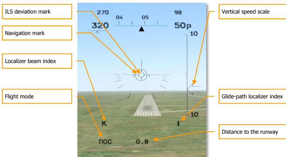
3-20: ILS landing
